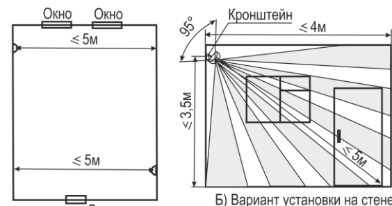
А) Вариант установки на стене (вид сверху)
